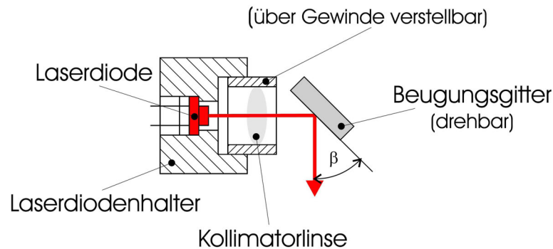
Abb. 4.4: Linienbreitenreduktion mittels Giterrückkopplung in Littrow-Konfiguration. Der von der Laserdiode emittierte Strahl wird kollimiert und trifft dann auf das Beugungsgitter. Die 1. Ordnung wird wieder zurück in die Diode reflektiert. Abb. entnommen aus [Unt05].
