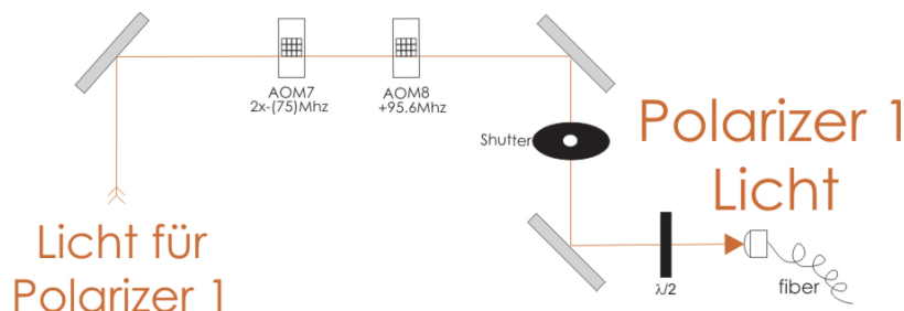
Abb. 5.14: Strahlverlauf des PL1-Lichts.
