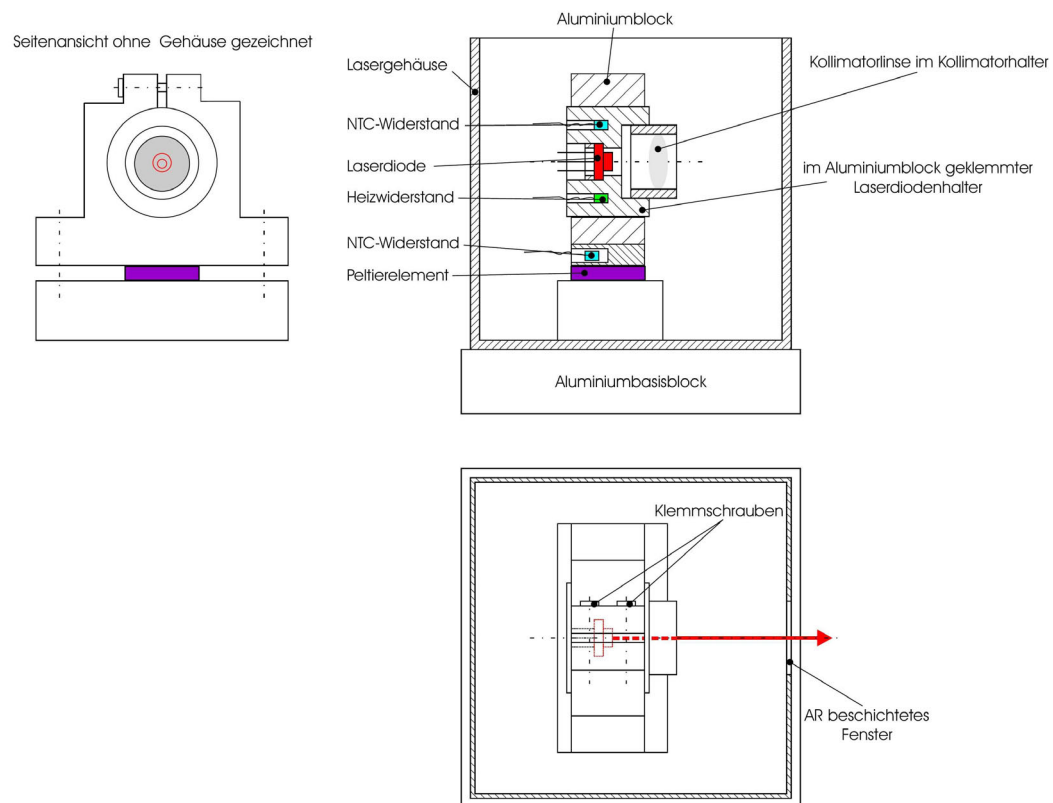
Abb. 4.6: Technischer Aufbau eines Slave-Lasers. Abb. entnommen aus [Unt05]
