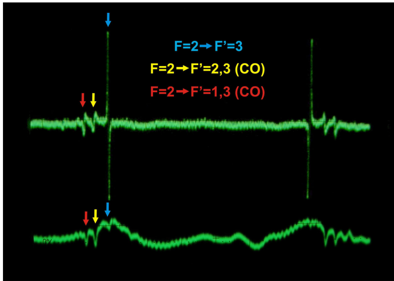
Abb. 5.4: Am Oszilloskop aufgenommenes Bild des Fehlersignals der Modulationstransfer-Spektroskopie (oben) samt Signal der zusätzlich zur Überwachung des Signals aufgebauten Sättigungs-Spektroskopie des ML1 (unten). Der ML1 wird auf den, im Bild mit dem blauen Pfeil markierten, Kühlübergang von F = 2 nach F' = 3 stabilisiert.
