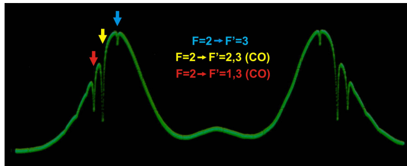
Abb. 5.11: Sättigungsspektroskopiesignal des Injektionslichtes für den Zeeman-Abbremser Slavelaser.
