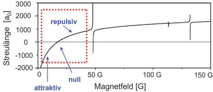
Abb. 2.3: Streulänge von ^{133}\text{Cs} im F = 3 , m_F = 3 Zustand abhängig vom angelegten Magnetfeld samt auftretender Feshbachresonanzen. Berücksichtigt werden nur Resonanzen, die sich aus einer Kopplung an Molekülzustände mit Bahndrehimpulsquantenzahl l = 0 bzw. l = 2 ergeben.
