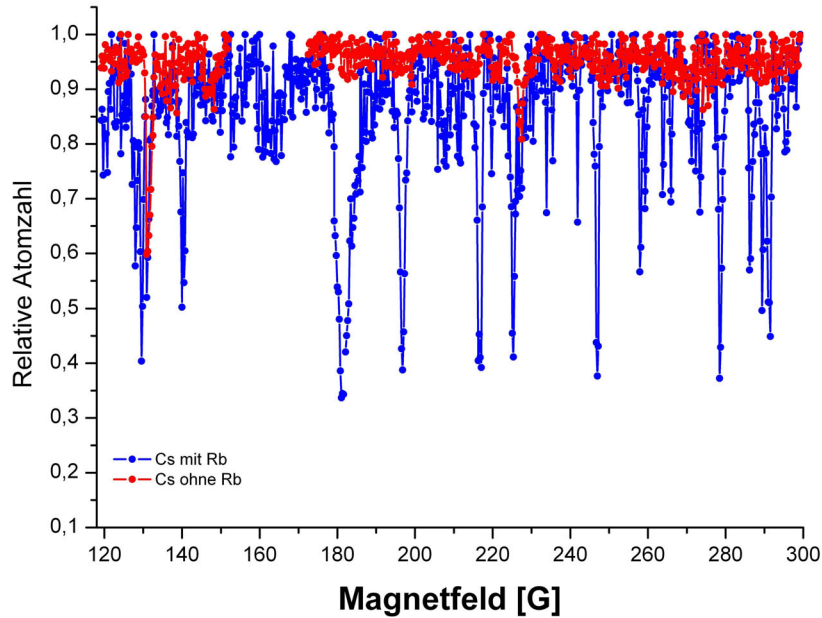
Abb. 6.3: Feshbach-Resonanzen für ^{133}\text{Cs} im F=3 , m_F=3 und für ^{87}\text{Rb} im F=1 , m_F=1 Zustand. Cs wird als Sonde für die, durch die Feshbachresonanzen verursachten, Dreikörperverluste verwendet. Für die roten Datenpunkte wurde nur Cs in die Falle geladen - die hierbei auftretenden Verluste entstehen durch reine Cs-Feshbachresonanzen. Sind gleichzeitig Rb-Atome anwesend (blaue Datenpunkte), so sind weitere Verluste zu erkennen, die auf RbCs-Interspezies-Feshbachresonanzen beruhen.
