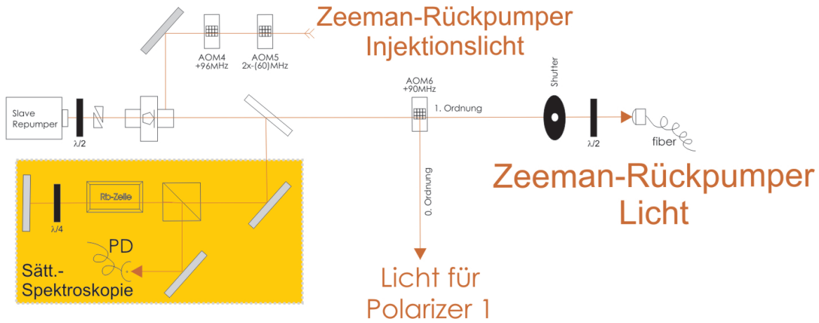
Abb. 5.12: Strahlverlauf des Zeeman-Rückpumpers.
