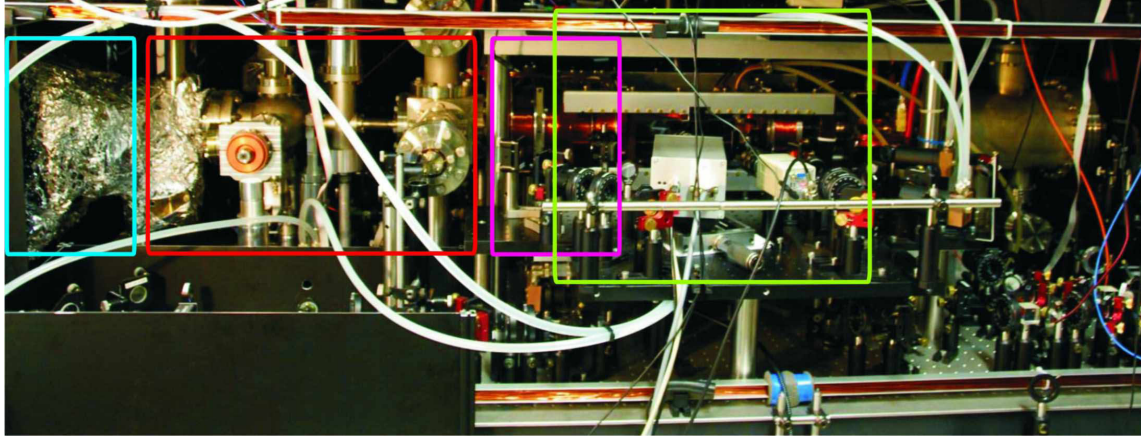
Doppelspeziesofen Differentielle Pumpstrecke Zeeman Abbremser Glaszelle&Magnetspulen
