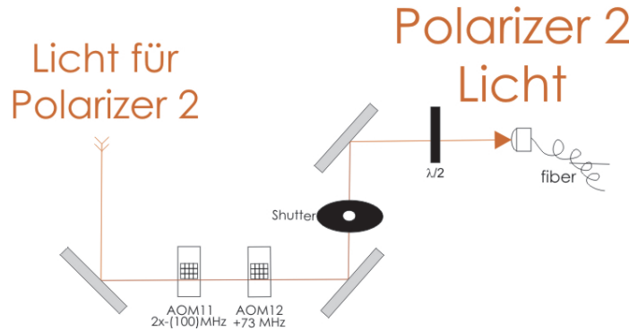
Abb. 5.15: Strahlverlauf des PL2-Lichts..
