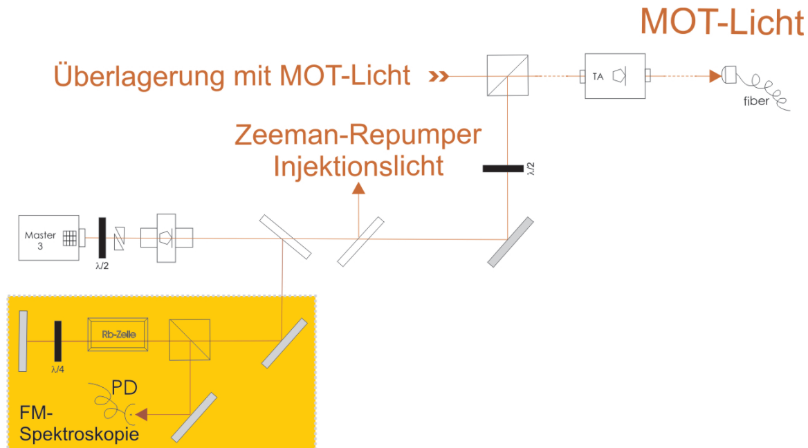
Abb. 5.7: Experimenteller Aufbau des MOT-Repumper Lasers.
