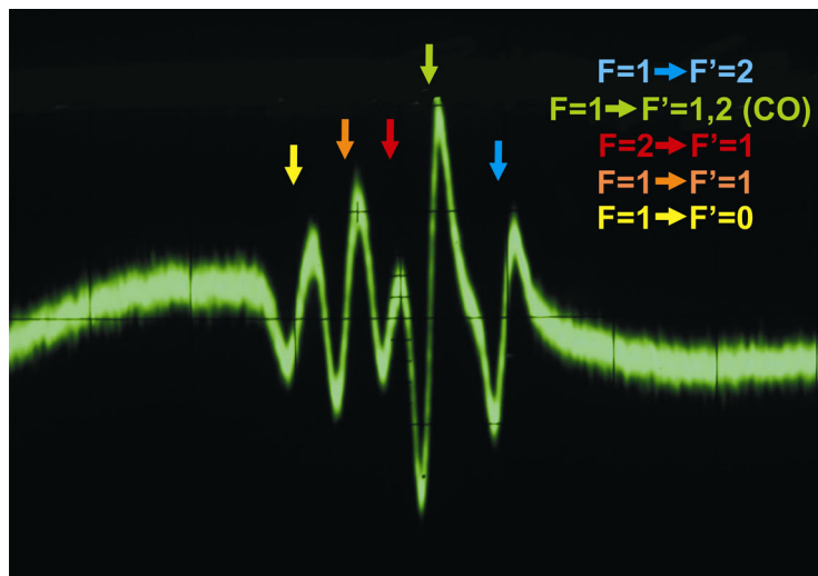
Abb. 5.9: Frequenzmodulations-Fehlersignal des ML3. Der Laser wird auf die steilste Flanke in der Mitte des Signals gelockt (im Bild mit einem grünen Pfeil markiert).
