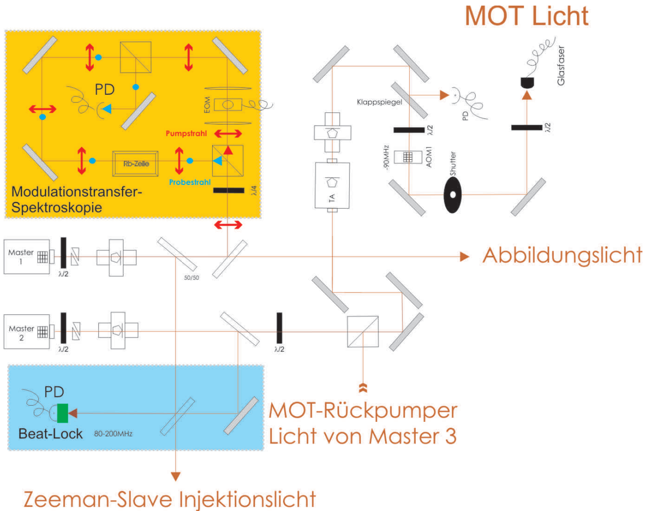
Abb. 5.2: Schematische Darstellung des MOT-Lasersystems.
