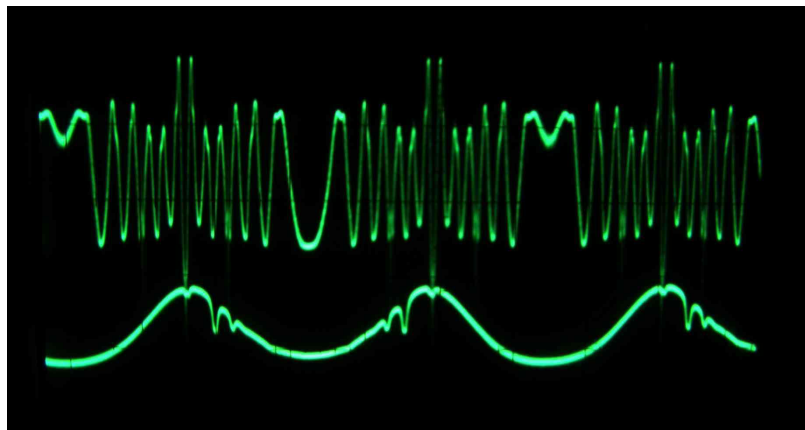
Abb. 5.6: Beat-Lock Signal (oben) samt Spektroskopiesignal des ML2 (unten).
