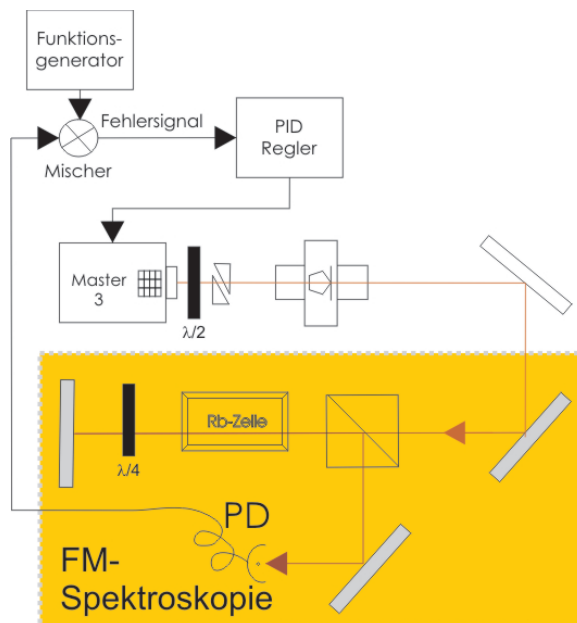
Abb. 5.8: Schematischer Überblick über den Aufbau der Frequenzmodulations-Spektroskopie. Dadurch, dass das Laserlicht über den Diodenstrom frequenzmoduliert wird, benötigt man keinen zusätzlichen EOM.
