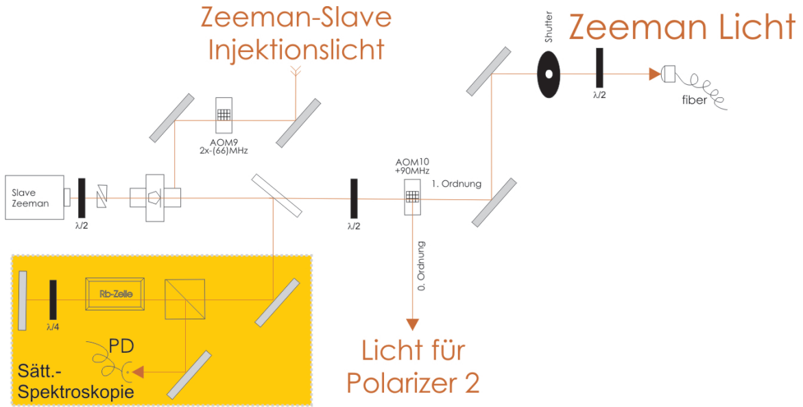
Abb. 5.10: Strahlverlauf des Zeeman-Abbremser-Lichts.
