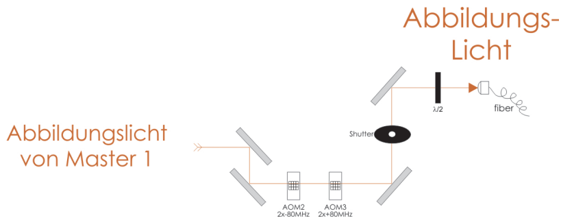
Abb. 5.16: Experimenteller Aufbau des Abbildungs-Strahls.
