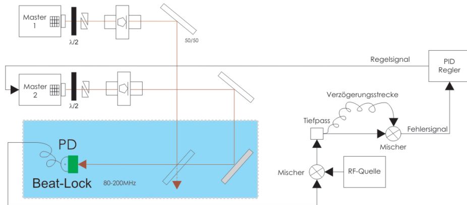
Abb. 5.5: Schematische Darstellung der Erzeugung des Beat-Signals und der dadurch erfolgenden Regelung des ML2.
