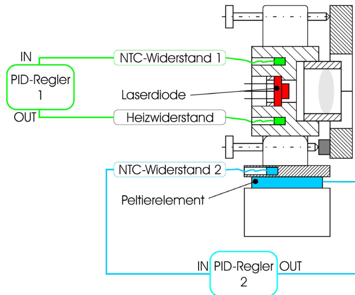
Abb. 4.3: Temperaturstabilisierung der Laserdiode. Die temperaturabhängigen Widerstände von NTC-Widerstand 1 und 2 werden in das Fehlersignal umgewandelt. Diese Signale werden anschließend von je einem PID-Regler in die Stellgröße umgesetzt. Über den Heizwiderstand (Regelkreis 1) und parallel über das Peltier-Element (Regelkreis 2) wird so die Temperatur der Diode geregelt. Abb. entnommen aus [Unt05].
