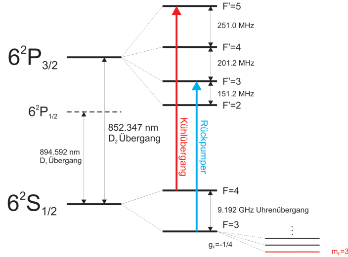
Abb. 2.1: Ausschnitt aus dem Termschema von ^{133}\text{Cs} . Schematisch sind die für die Laserkühlung benötigten Übergänge eingezeichnet.
