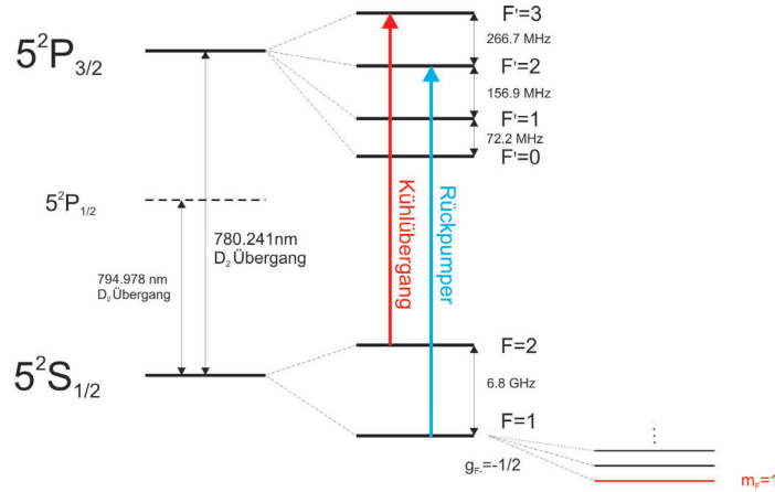
Abb. 2.2: Ausschnitt aus dem Termschema von ^{87}\text{Rb} . Schematisch sind die für die Laserkühlung benötigten Übergänge eingezeichnet.
