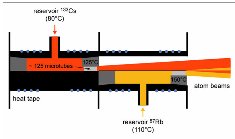
Abb. 2.6: Schematischer Aufbau des neuen Doppelspeziesofens.
